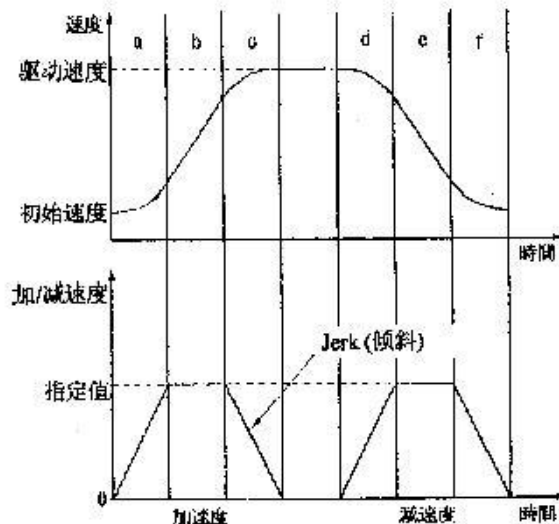
图 2.2.7 S 曲线加减速驱动
