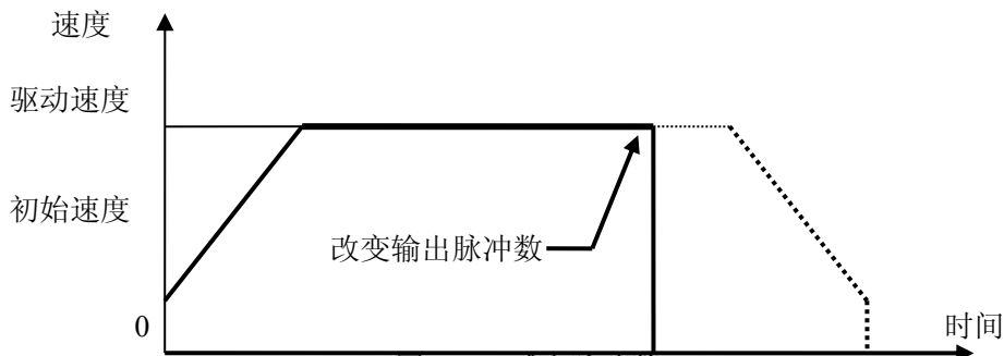
图 2.1.4 减少脉冲数
