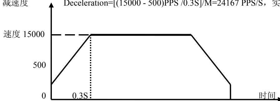
图 2.2.3 定长脉冲驱动模式
