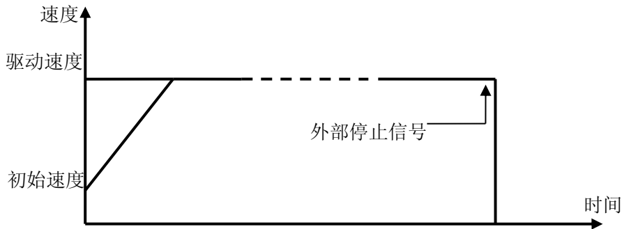
图 2.1.6 连续脉冲驱动
