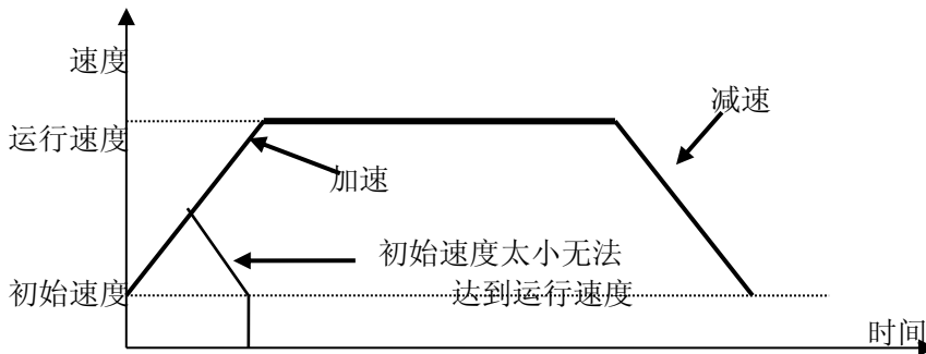
图 2.2.2 直线加/减速
