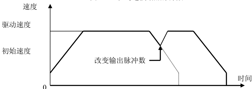
图 2.1.3 在降速段增加脉冲数
