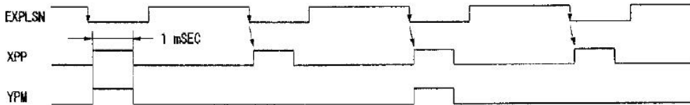
图 2.4.6 根据外部信号(EXPLSN)的步进插补例子(驱动速度: 500PPS)
